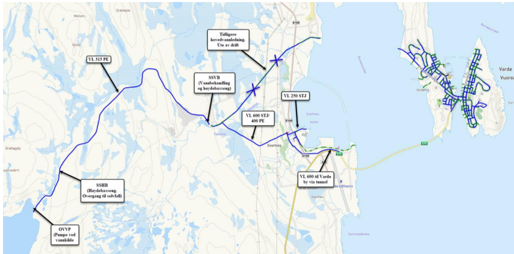
Figur 37: Utklipp av Vardø kommune sitt digitale kartløsning med VA-anlegg med påskrevne kommentarer.
